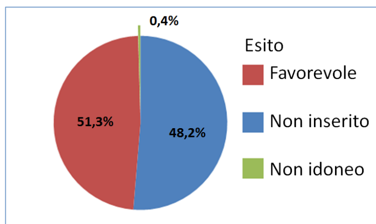
Figura 2: dati riferiti a 2484 campioni caricati sul sistema SINVSA da gennaio ad ottobre 2020 relativamente agli esiti dei test di laboratorio nell'ambito della sorveglianza passiva per PSA.
