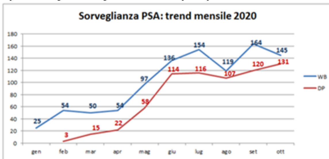
Fig. 1: andamento mensile dei dati di sorveglianza passiva per PSA caricati su SINVSA distinto per suini domestici (DP) e cinghiali (WB) da gennaio a ottobre 2020.
